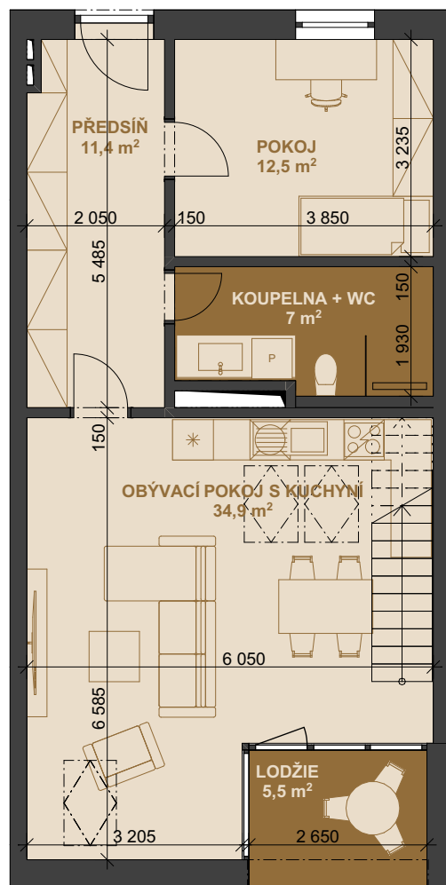
Půdorys 3.NP
