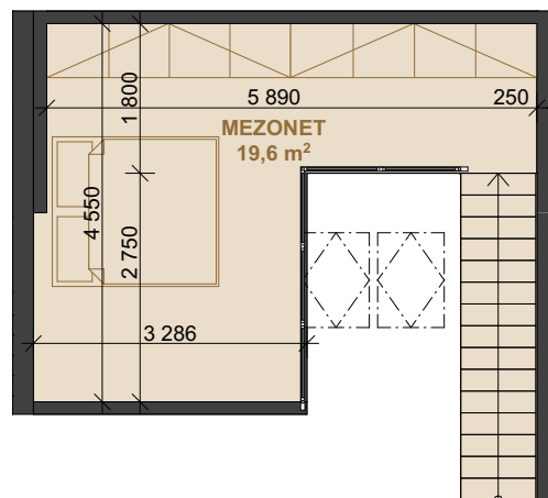
Půdorys 4.NP - mezonet
